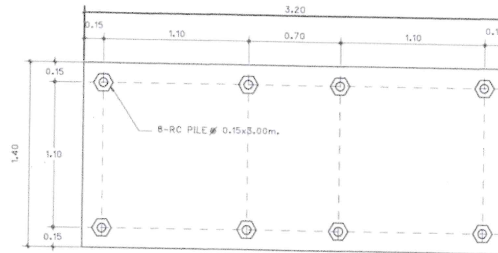
แปลนฐานราก TYPE II
