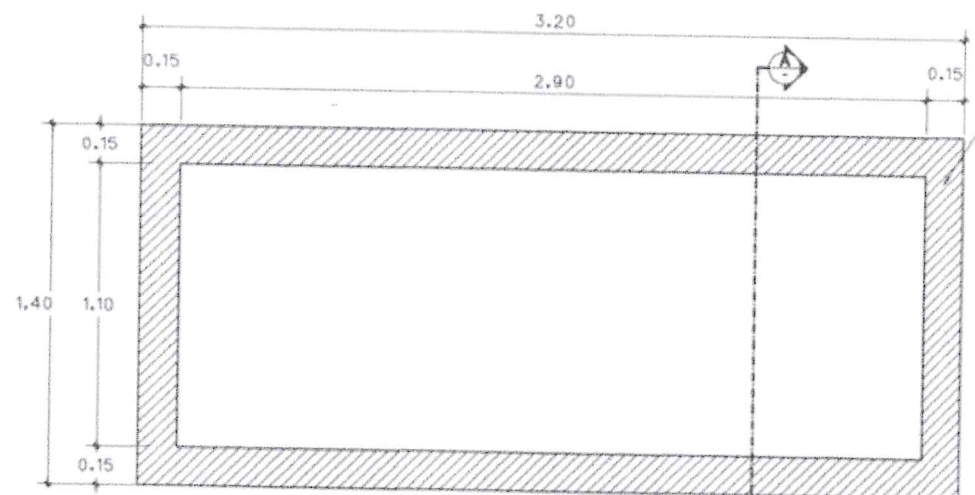
แปลนฐานอุปกรณ์
